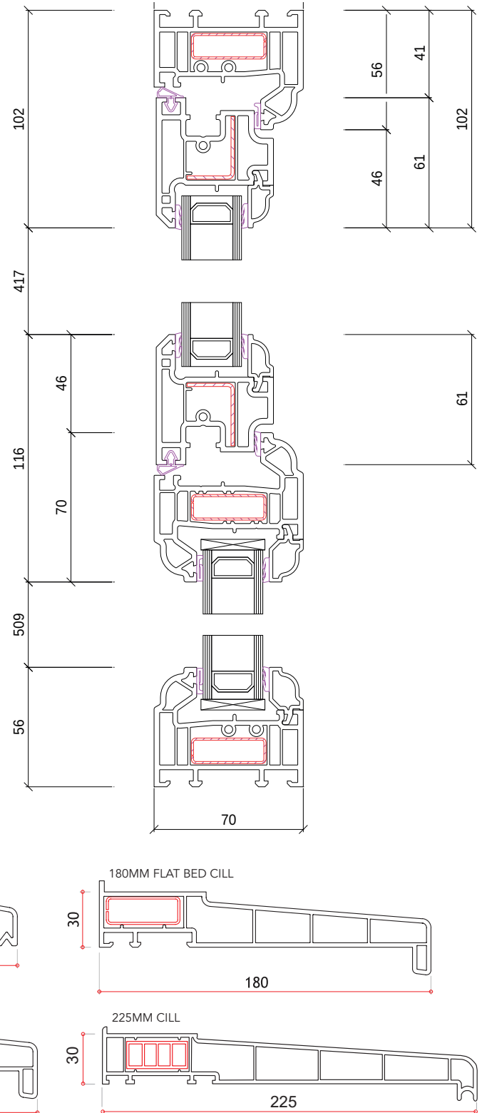
Rustique Flush Sash (ovolo)
